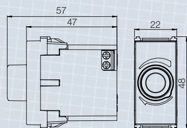
Módulo dimmer
