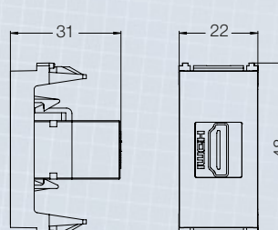
Módulo HDMI
