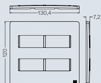
Placa 4x4 4 POS
