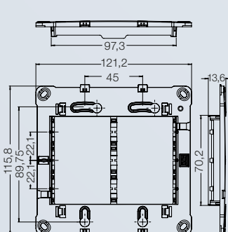
Suporte 4x4
