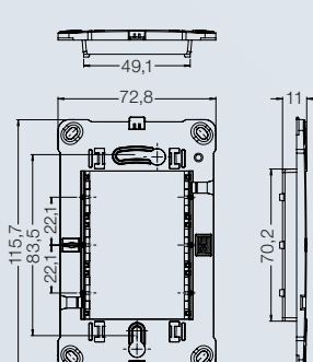
Suporte 4x2
