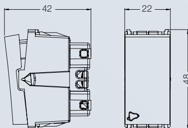
Pulsador campainha
