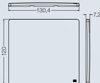
Placa 4x4 CEGA
