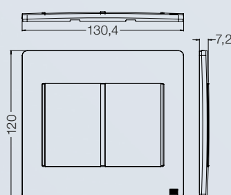
Placa 4x4 6 POS
