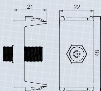
Módulo antena
