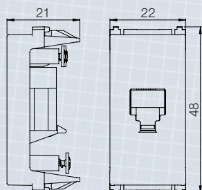
Módulo RJ11
