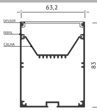
Desenho Técnico
