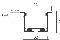
Desenho Técnico
