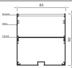
Desenho Técnico
