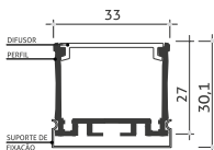
Desenho Técnico
