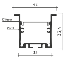
Desenho Técnico
