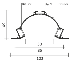
Desenho Técnico
