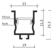
Desenho Técnico
