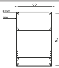
Desenho Técnico
