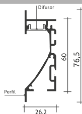
Desenho Técnico
