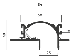
Desenho Técnico
