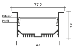
Desenho Técnico
