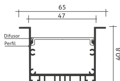
Desenho Técnico
