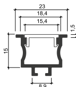
Desenho Técnico
