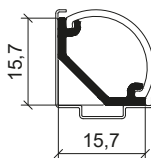
Desenho Técnico
