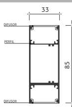
Desenho Técnico
