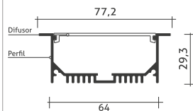
Desenho Técnico
