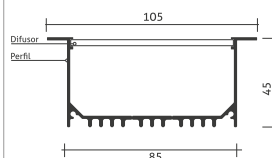
Desenho Técnico
