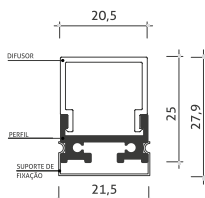
Desenho Técnico
