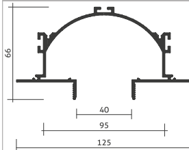
Desenho Técnico
