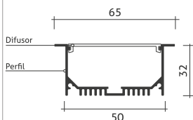
Desenho Técnico
