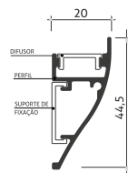
Desenho Técnico
