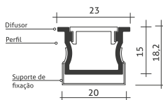
Desenho Técnico
