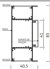
Desenho Técnico
