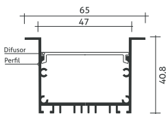
Desenho Técnico
