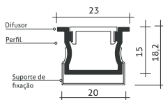
Desenho Técnico
