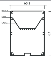
Desenho Técnico
