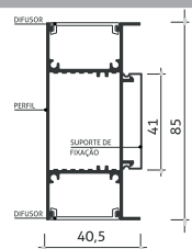
Desenho Técnico
