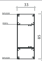
Desenho Técnico
