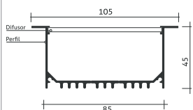
Desenho Técnico
