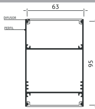
Desenho Técnico
