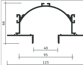
Desenho Técnico
