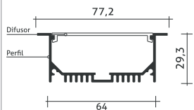
Desenho Técnico
