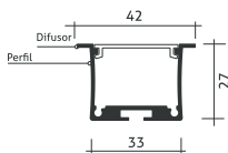
Desenho Técnico
