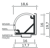
Desenho Técnico
