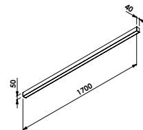
PL40002LED
