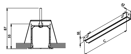
SISTEMA LINEAR EMBUTIR NEW FIT40
