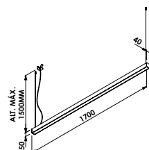
PD40002LED
