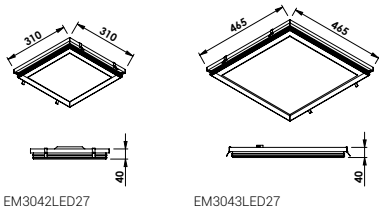
EM3042LED27
