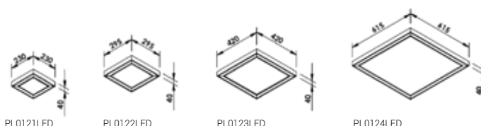
PL0121LED
