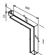
CURVA EMBUTIR TETO/PAREDE NEW FIT40
