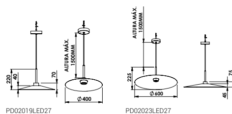
PD02019LED27
